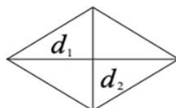
Ромб
