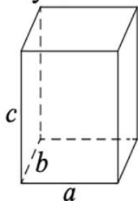
Прямоугольный параллелепипед
