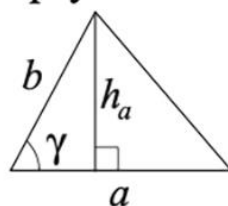
Треугольник
