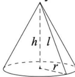
Конус
