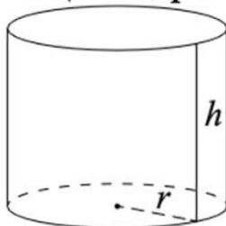
Цилиндр
