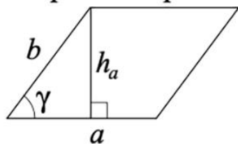
Параллелограмм
