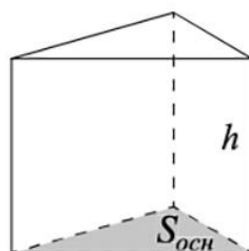
Прямая призма
