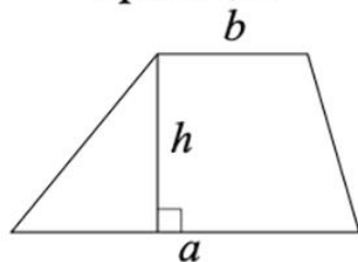
Трапеция
