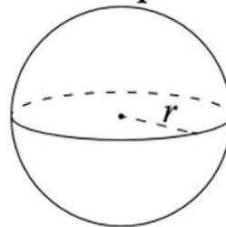
Шар
