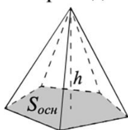
Пирамида
